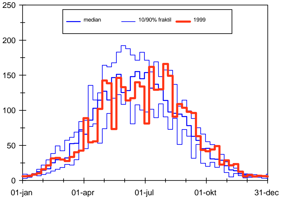
Figur 2.3: Globalstråling ved Hornum 1999 (ugesum)
