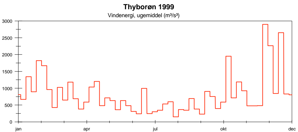
Figur 2.6: Vindhastighed, - retning og - energi ved Thyborøn 1999 (ugemiddel)
