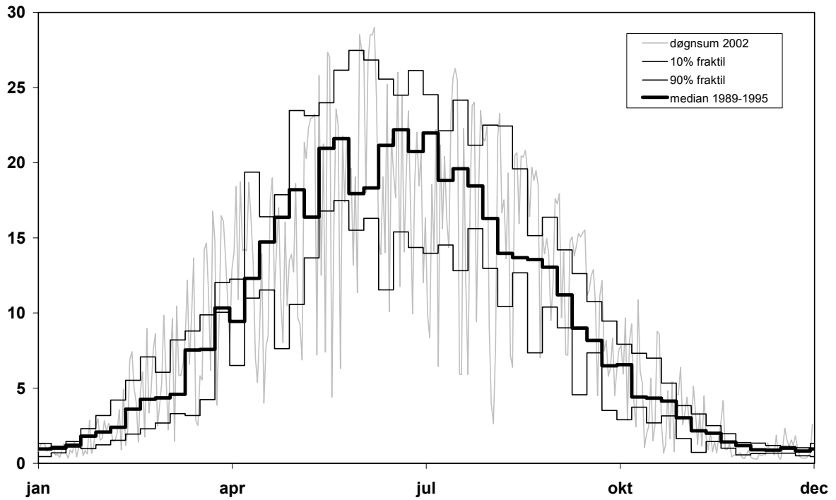
Bilag 2. Figur 2.11: globalstråling ved Hornum/Års 2002 (Vesthimmerland).
