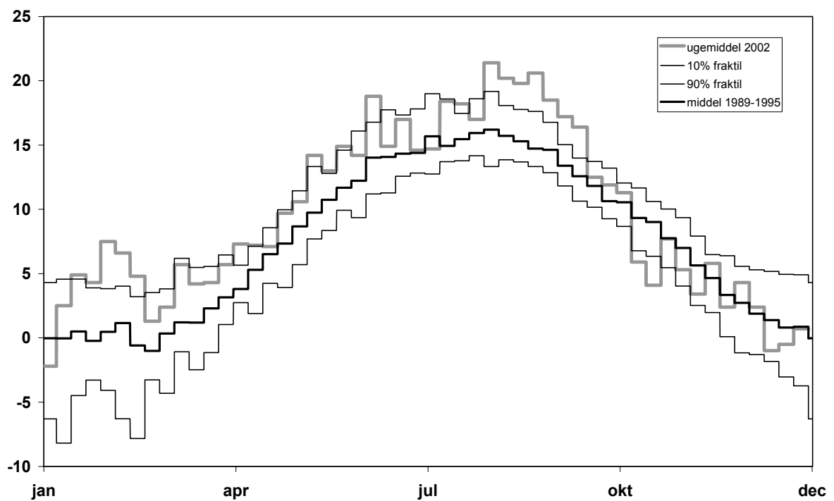
Bilag2. Figur 2.12: Lufttemperatur ved Aalborg Lufthavn 2002.
