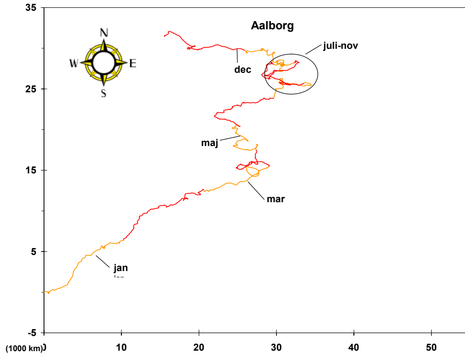
Bilag 2. Figur 2.6: Vindvektordiagram for Aalborg Lufthavn 2002 (km).
