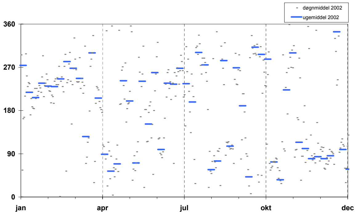
Bilag 2. Figur 2.7-9: vindhastighed, -retning og -energi ved Thyborøn 2002.
