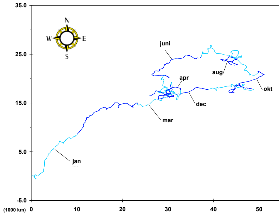
Bilag 2. Figur 2.10: Vindvektordiagram for Thyborøn 2002 (km)
