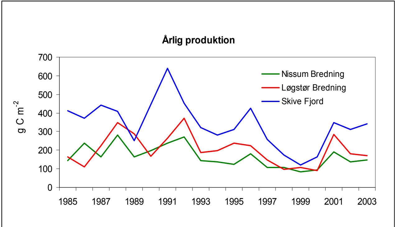
Primærproduktionen af fytoplankton i Nissum Bredning, Løgstør Bredning og Skive Fjord fra 1985-2003, årsmidler.
