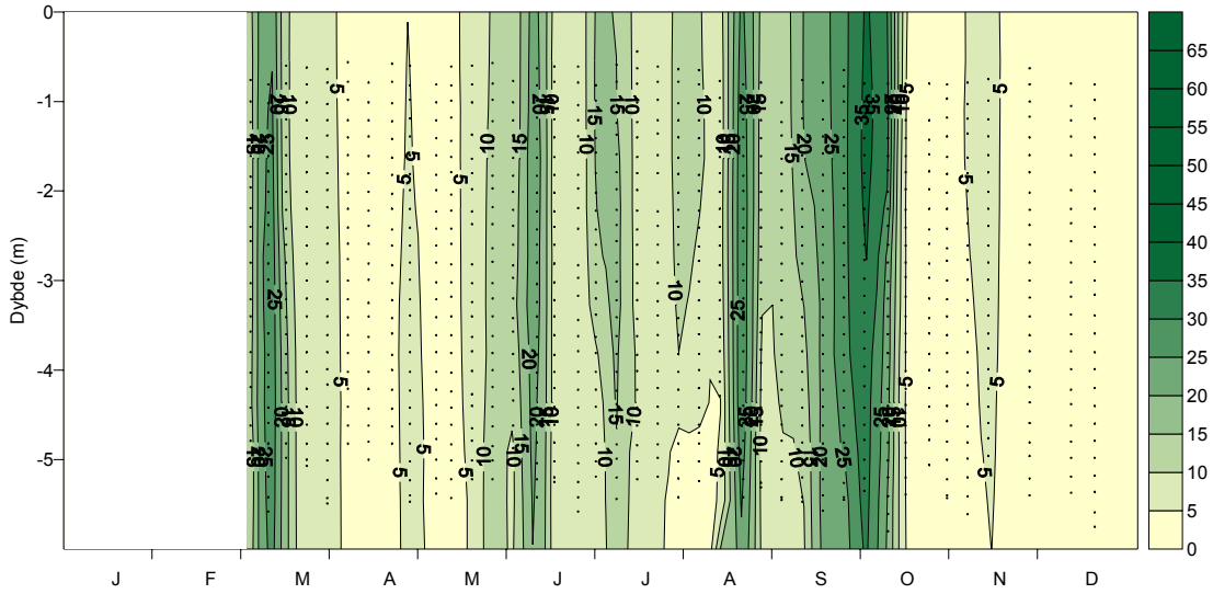
Fluorescensprofil - Nibe Bredning 2003
