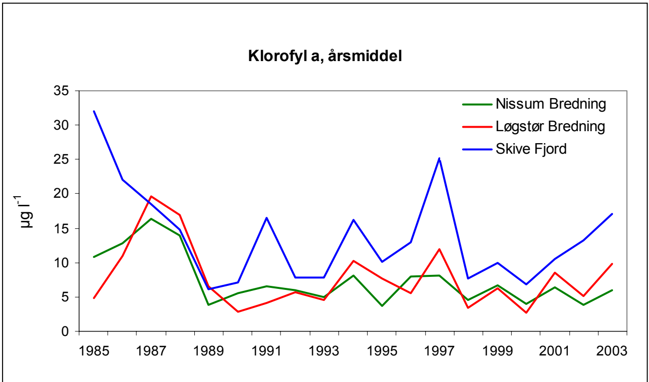
Koncentrationen af klorofyl a i Nissum Bredning, Løgstør Bredning og Skive Fjord fra 1985-2003, årsmidler.
