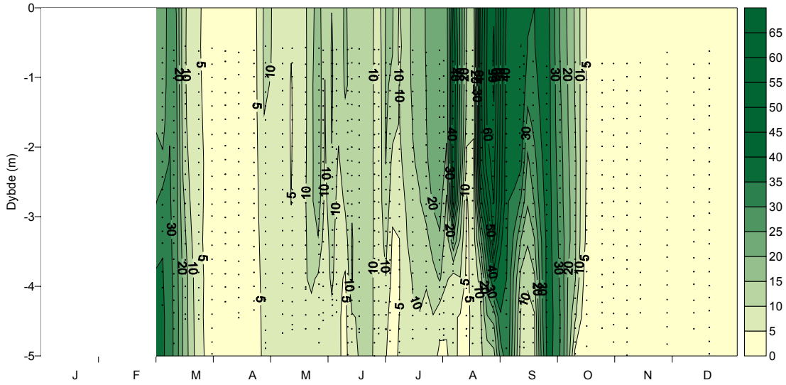
Fluorescensprofil - Lovns Bredning 2003
